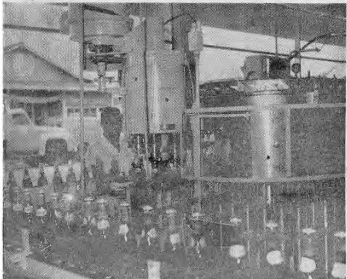
Fases parciales del embotellamiento de Pepsi Cola. Esta maquinaria de 28 válvulas es la más moderna de Centro América. 100 botellas por minuto
